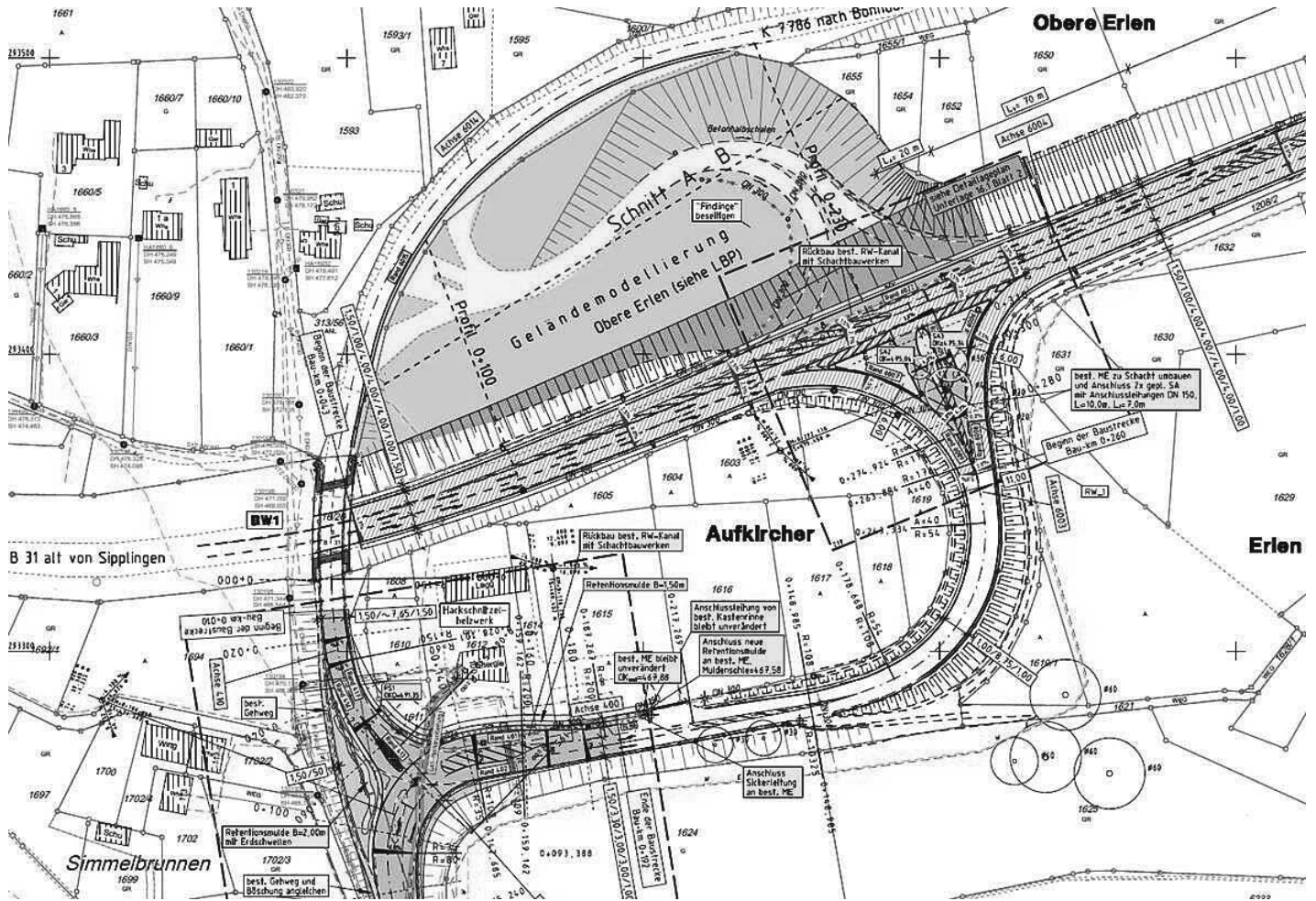
Lageplan zu den Umbauarbeiten am Knoten B 31alt/K 7786 bei Überlingen-Aufkirch
